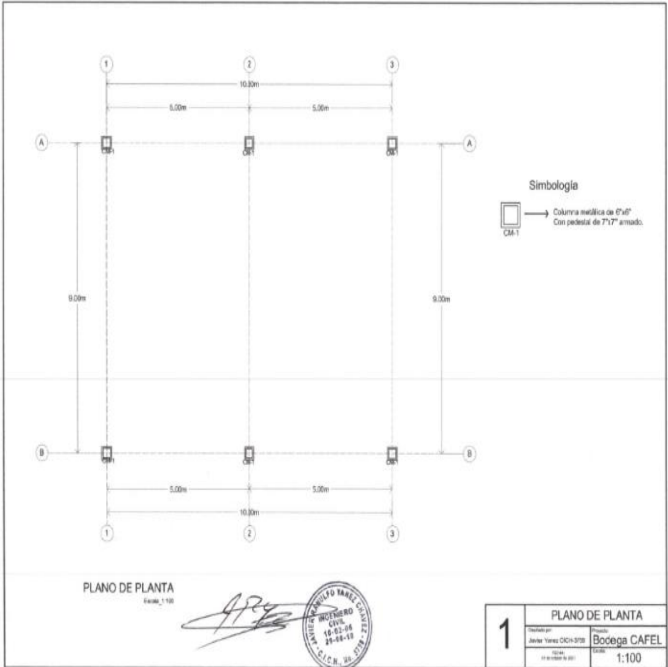
Plano No. 1. Planta de Cubierta de Techo
