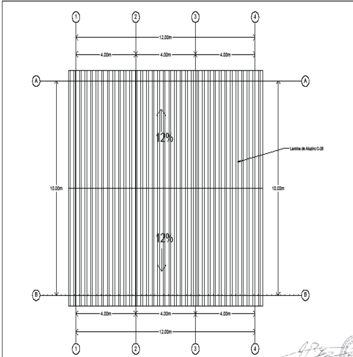
PLANO DE TECHO Escala: 1/100
