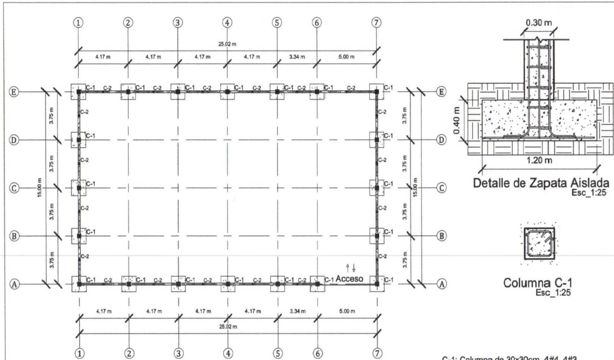
Plano de Estructura Esc_1:200
