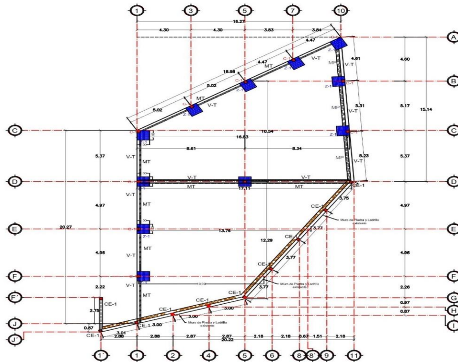
PLANO 1: Planta de Cimentación.
