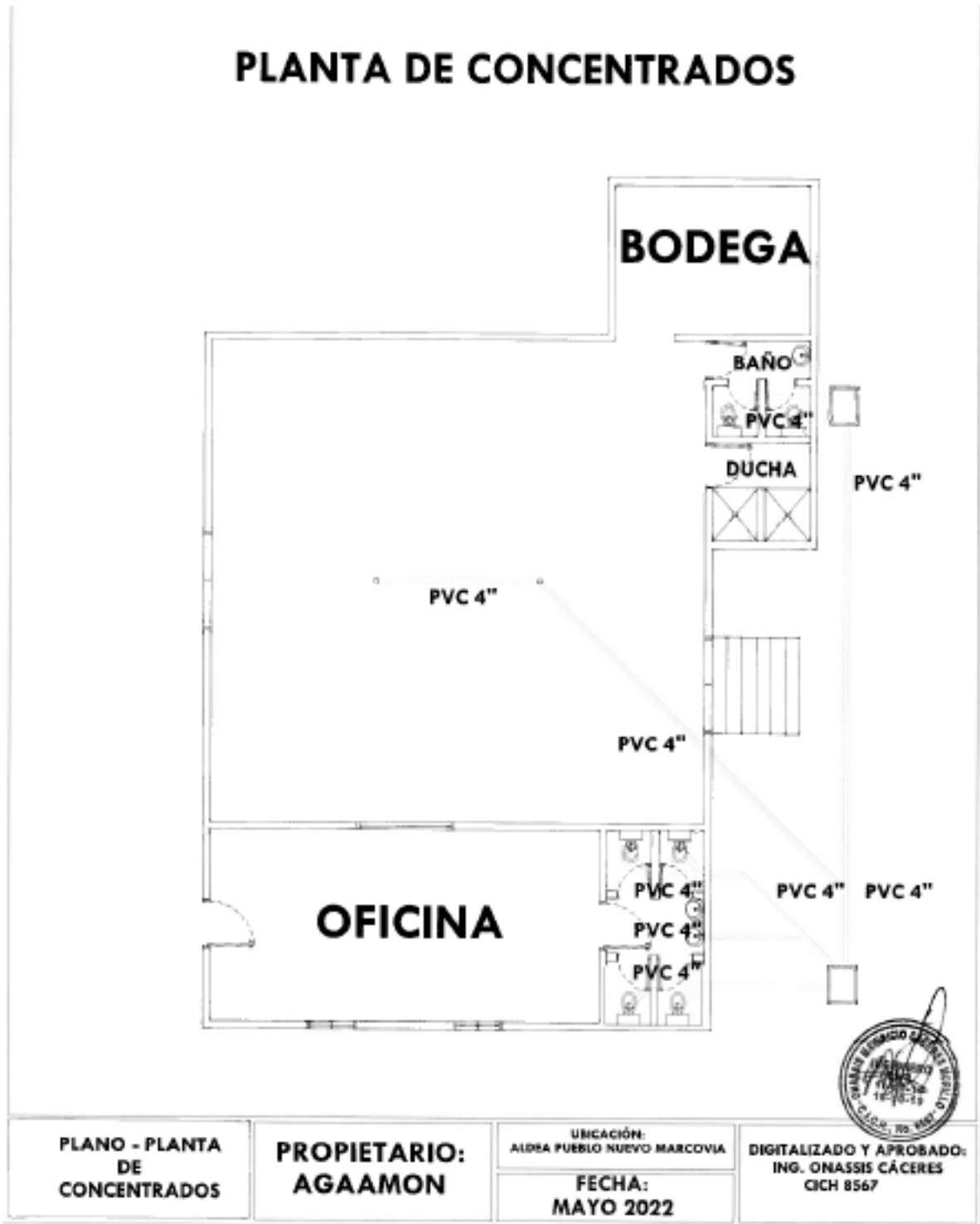
Plano No. 4 Plano hidrosanitario (Drenajes)
