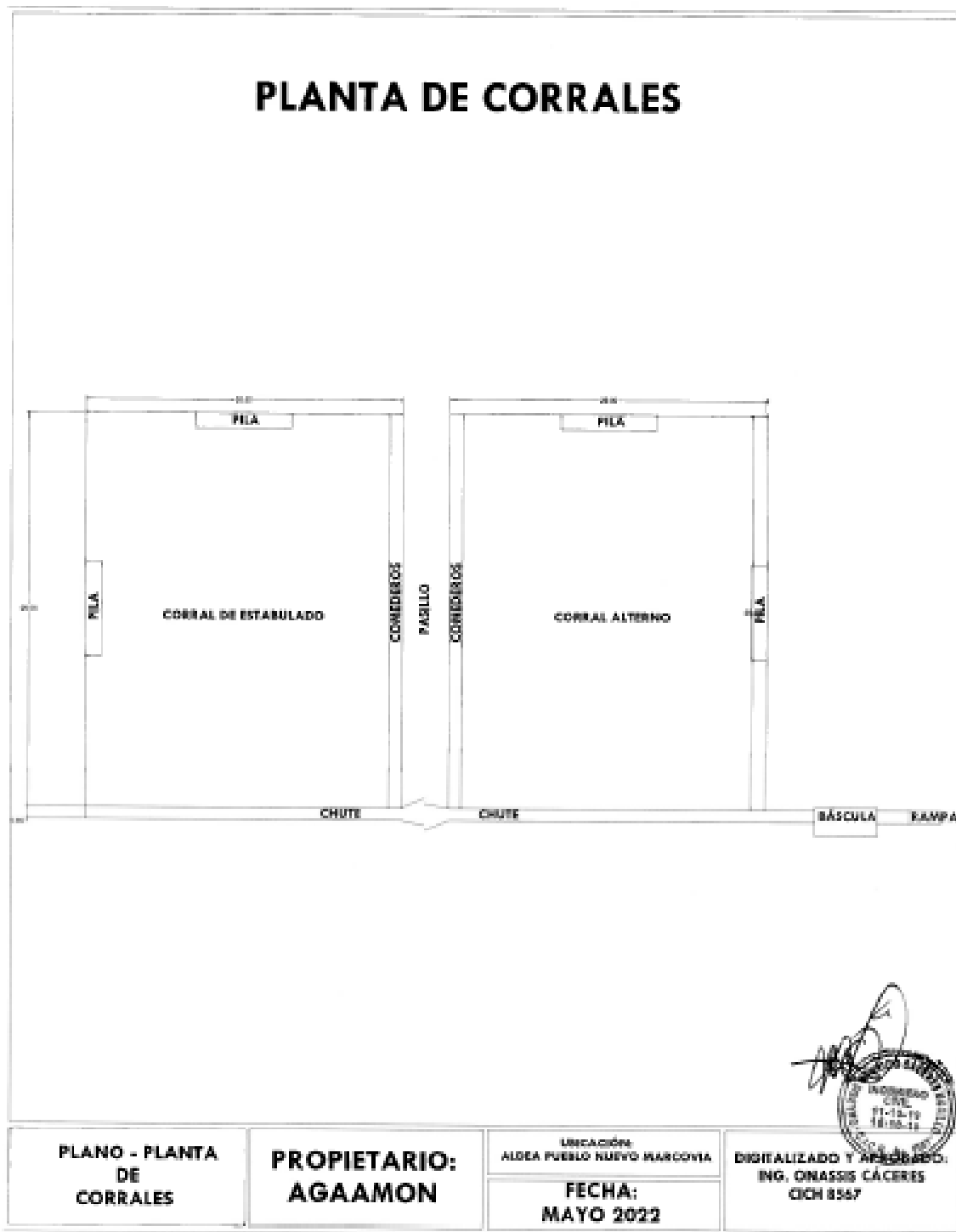
Plano No. 1 Plano Planta Arquitectonica
