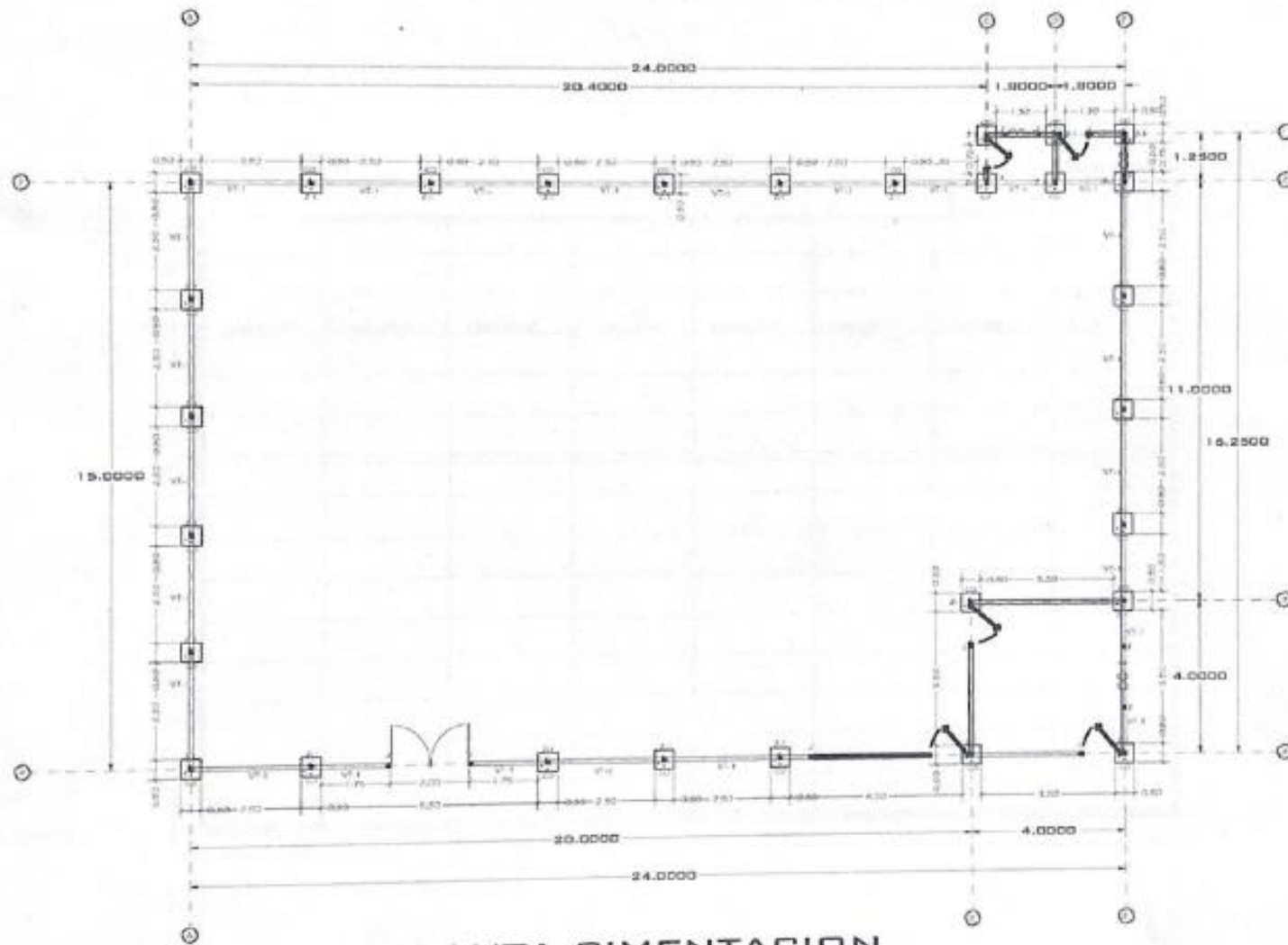
PLANTA CIMENTACION
