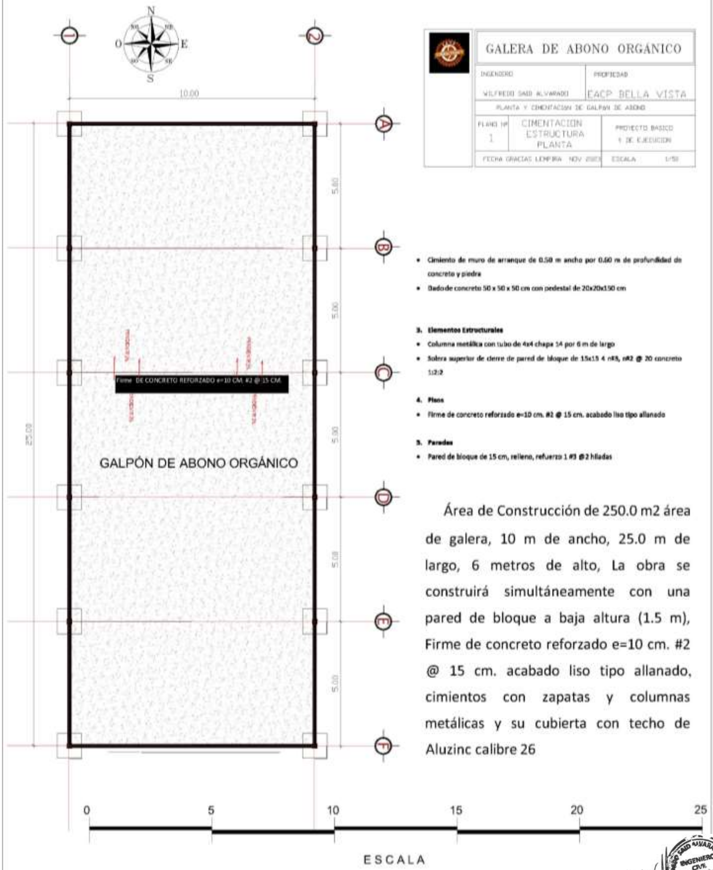
Plano No. 1 Infraestructura para la elaboración de abonos orgánicos
