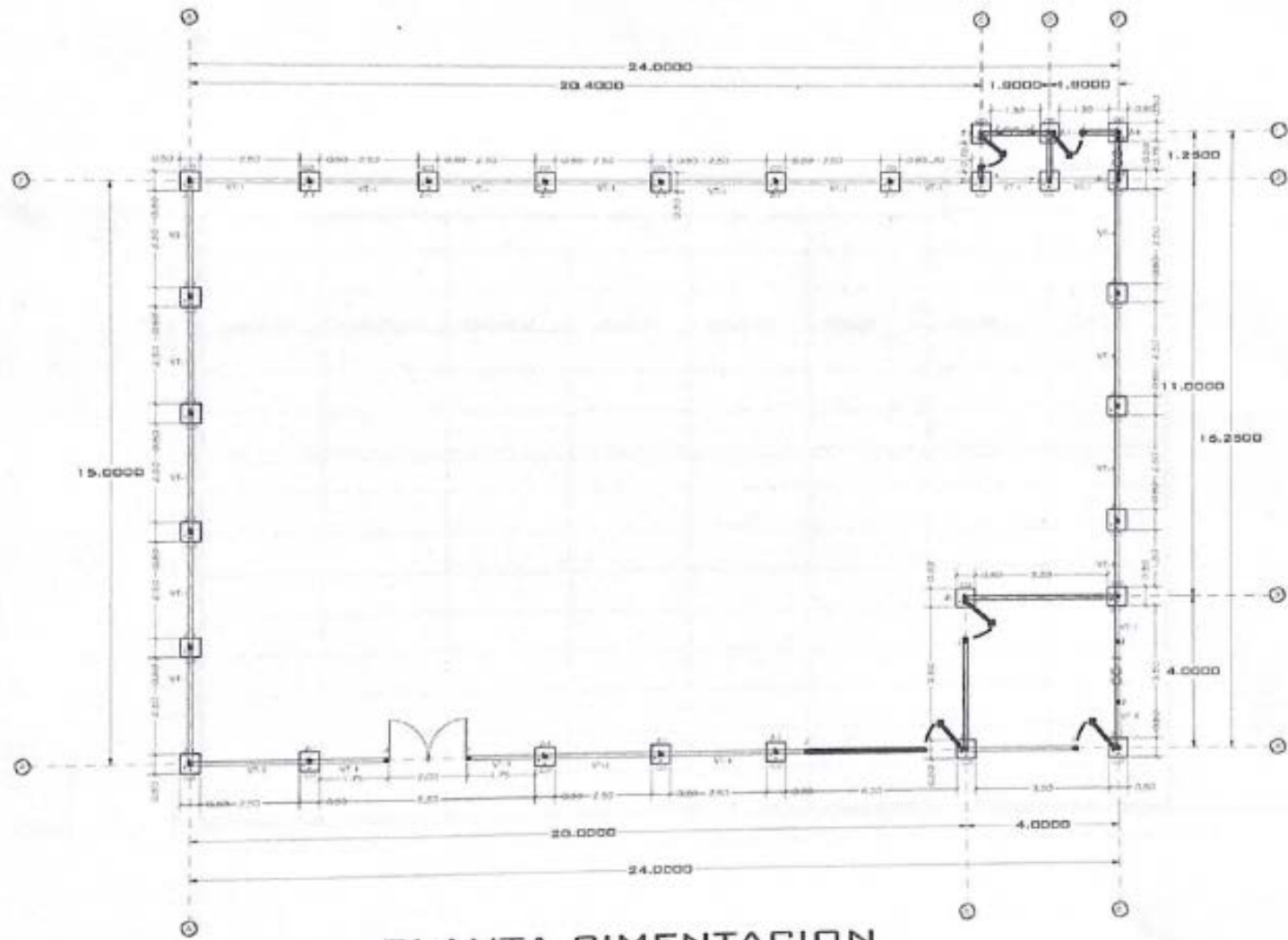
PLANTA CIMENTACION
